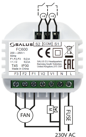
V1: Клапан нагрева/охлаждения V2: Не доступно
