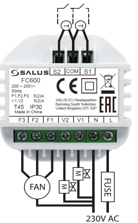
V1: Клапан нагрева V2: Клапан охлаждения
