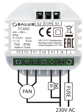
V1: Клапан нагрева/охлаждения V2: Не доступно
