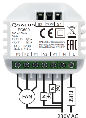
V1: Клапан нагрева V2: Клапан охлаждения
